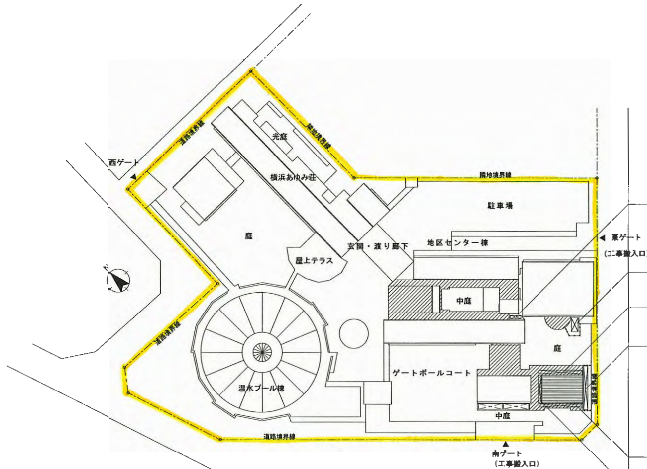
配置兼仮設参考図 1/1000
