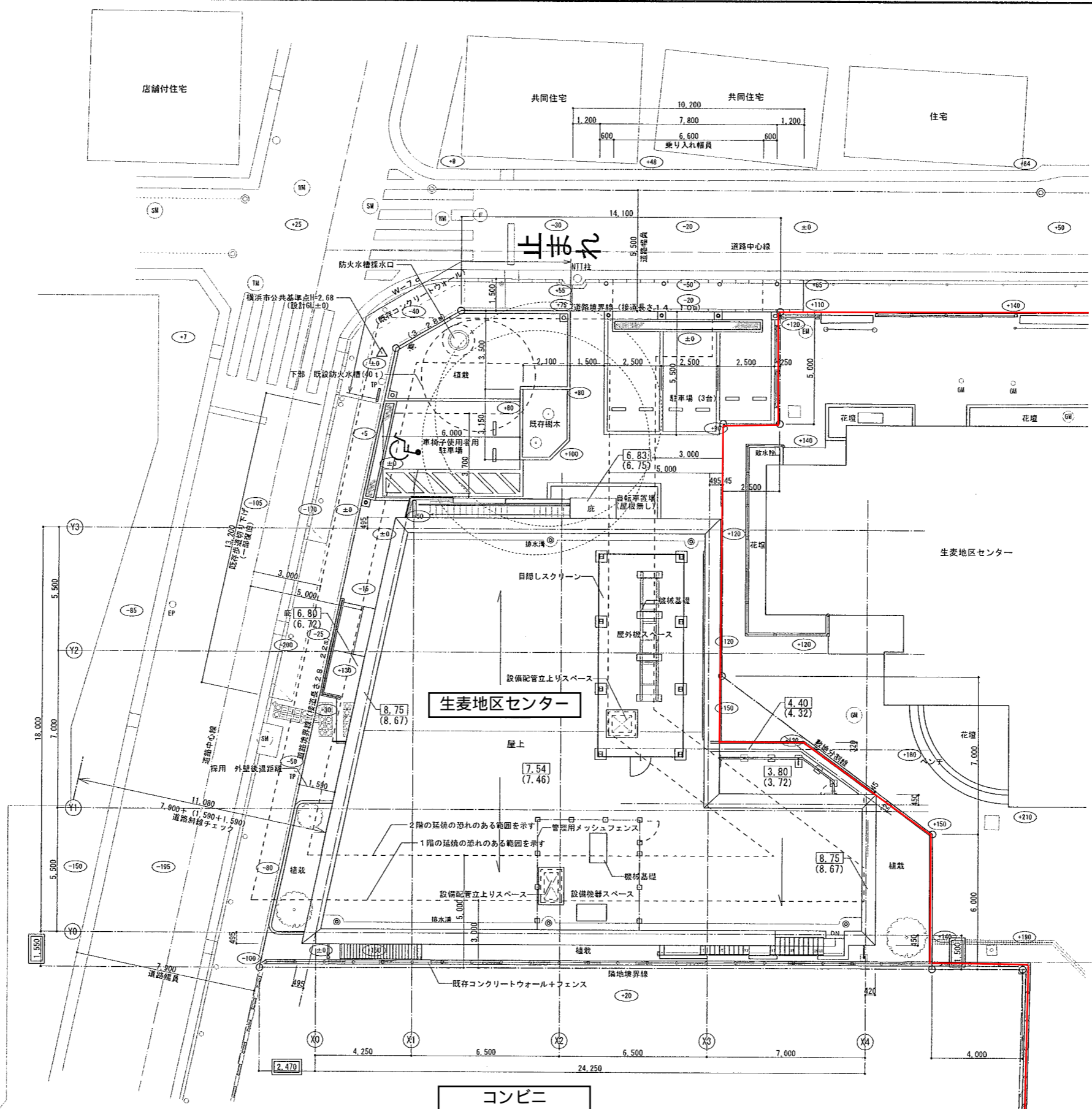
配置図 縮尺1/100
