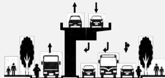
目黒交番前交差点立体化 (幅員25m)
