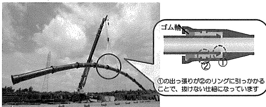
耐震管
