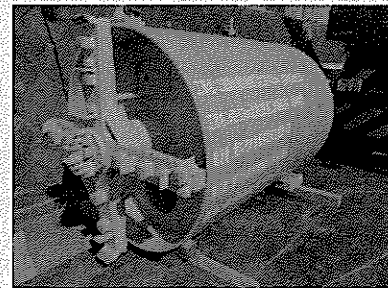
地下にトンネルを掘る機械 （推進機 外径 1600mm）
