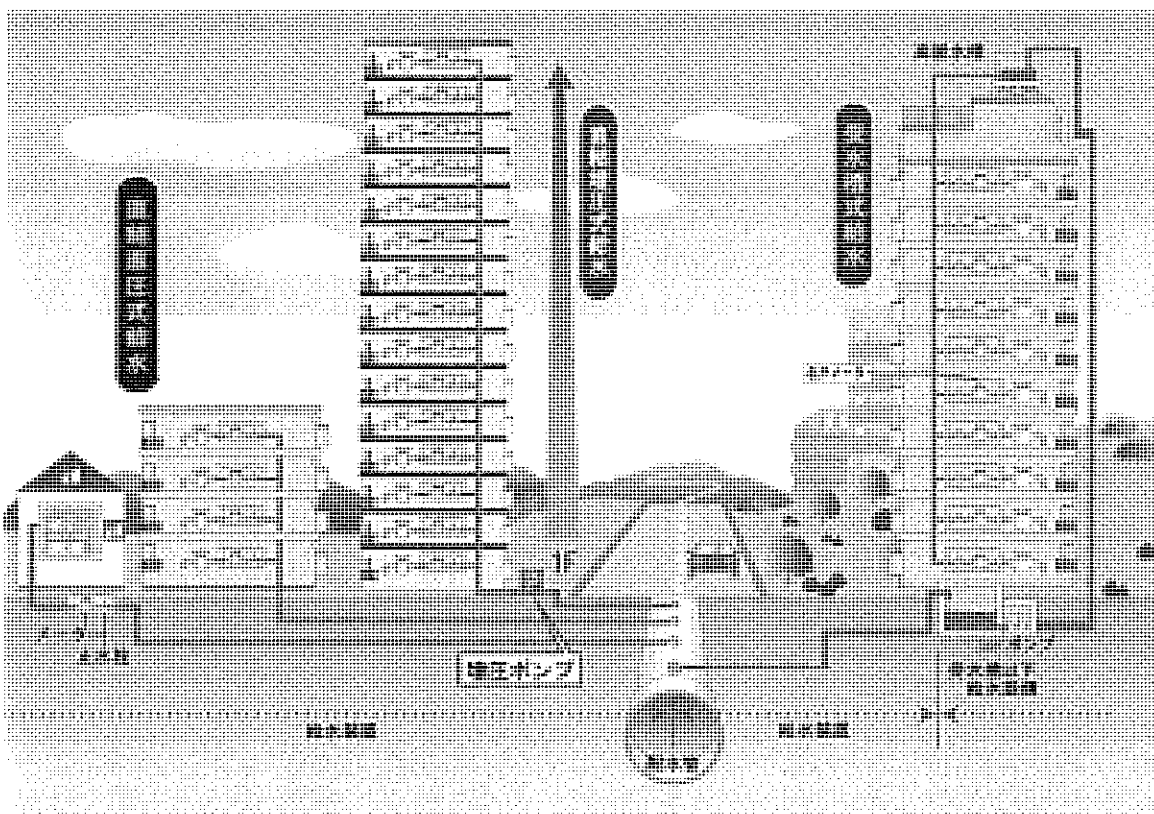
給水方式の種類
