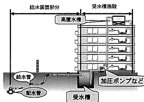
給水装置と受水槽施設の範囲
