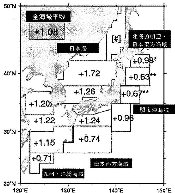
図 1-3 日本近海の海域平均海面水温（年平均）の変化傾向（℃/100 年）
