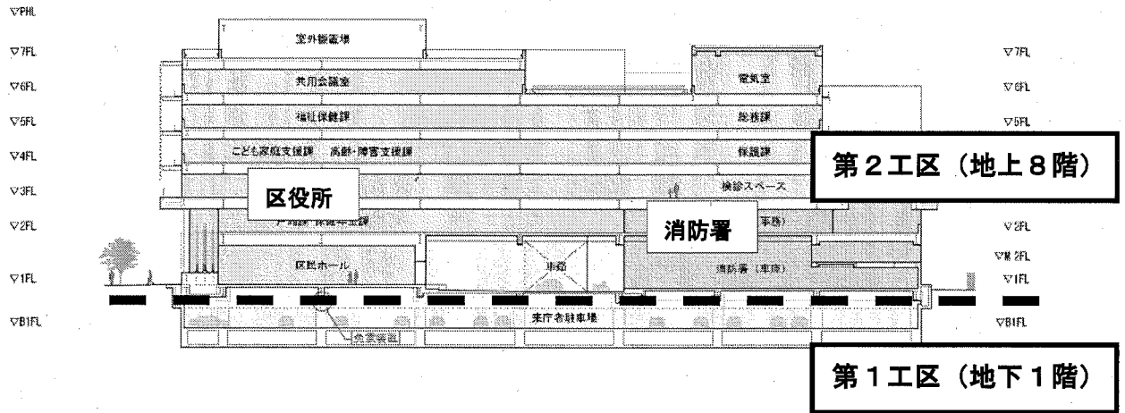
建物断面図
