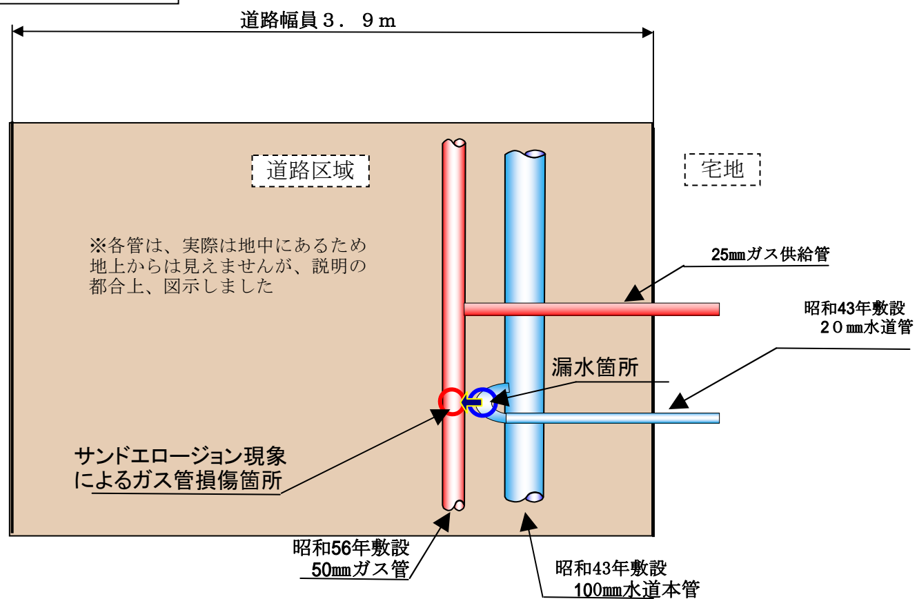
平面図
