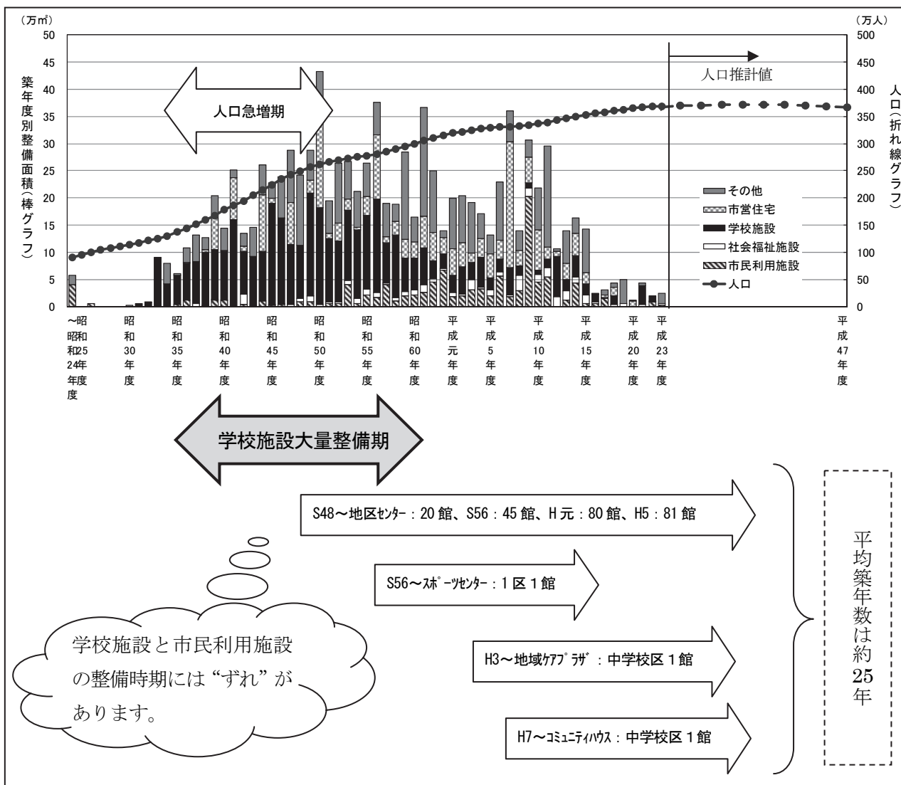
図 公共建築物の築年度別整備状況
