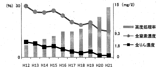
高度処理の導入と処理水に含まれる全窒素・全りん濃度の推移
