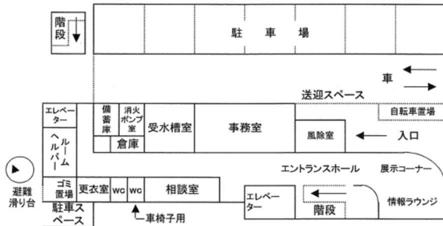
1階平面図
