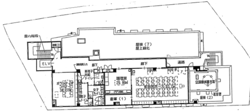
3階平面図
