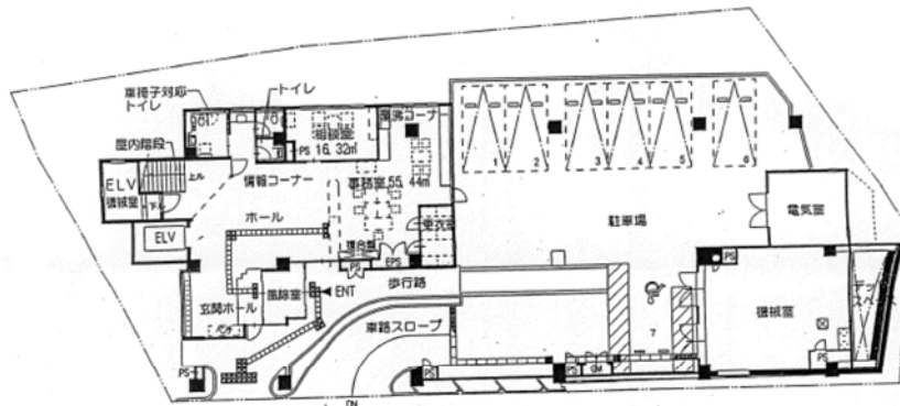
1階平面図
