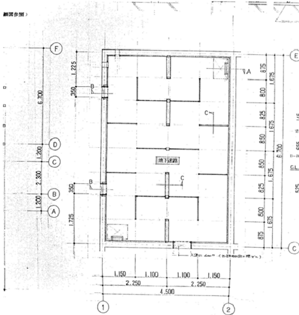
地下通路平面詳細図 S1/50
