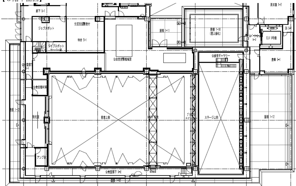
【5階平面図】
