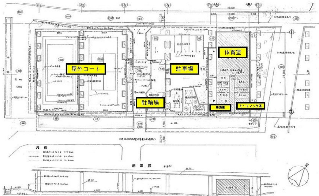
十日市場スポーツ会館平面図（その1 配置図）
