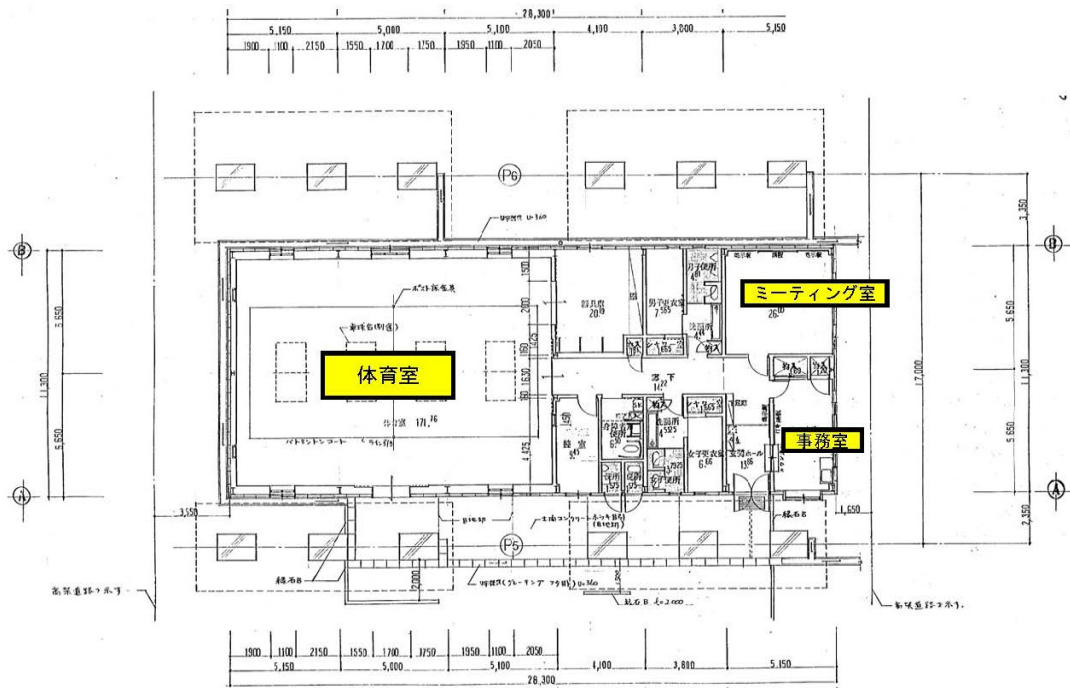
十日市場スポーツ会館平面図（屋内平面図）
