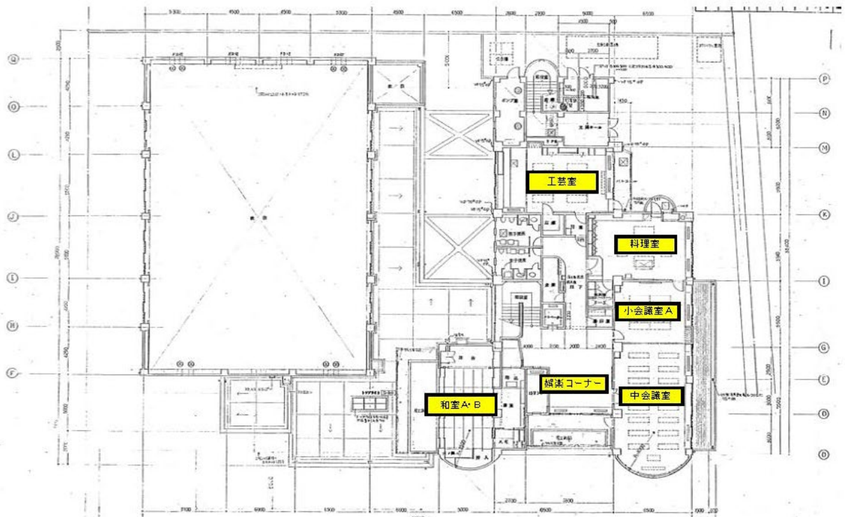
十日市場地区センター平面図（2階）
