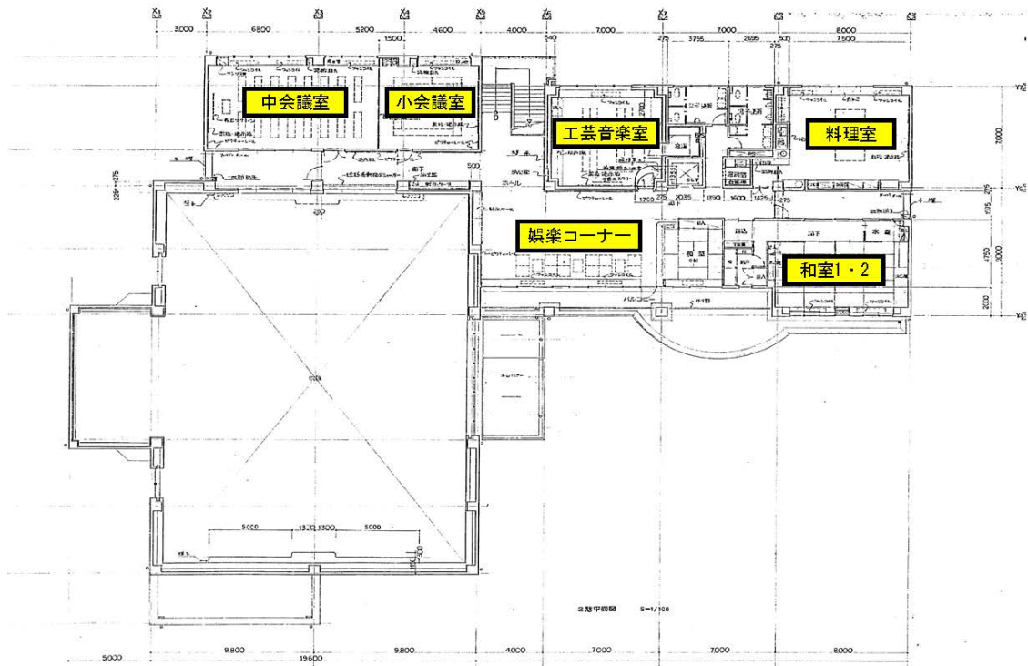
白山地区センター平面図（2階）
