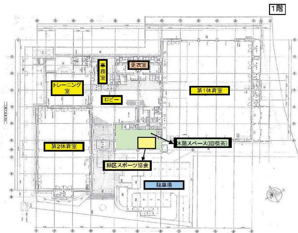
緑スポーツセンター平面図
