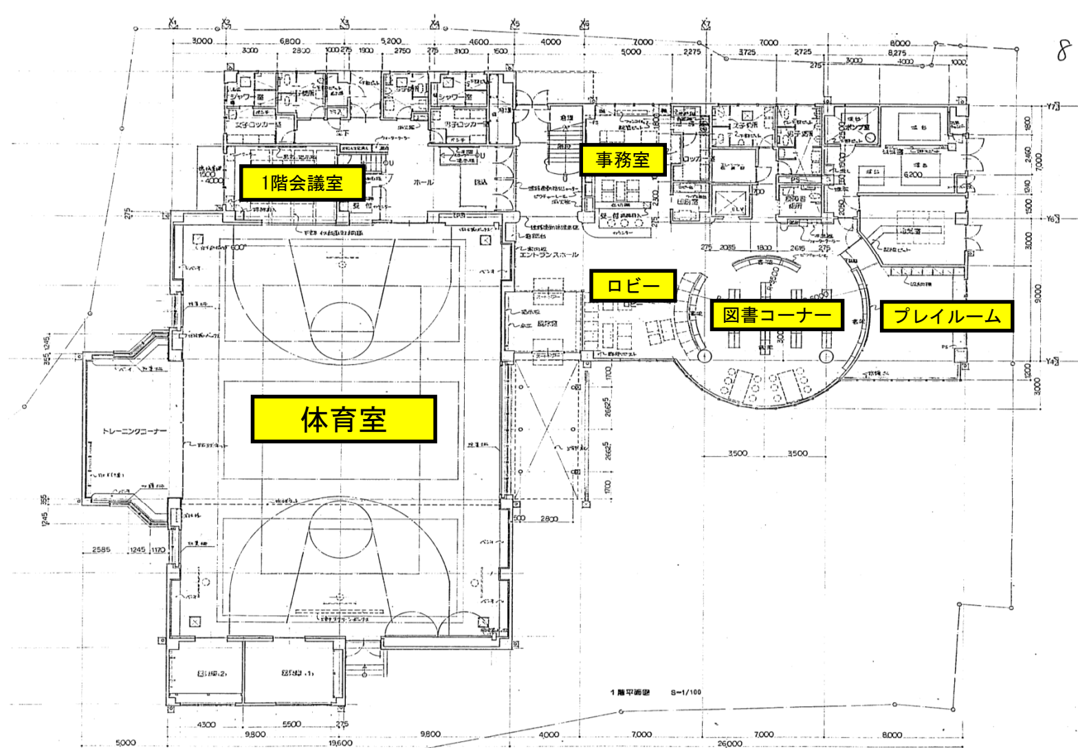
白山地区センター平面図（1階）
