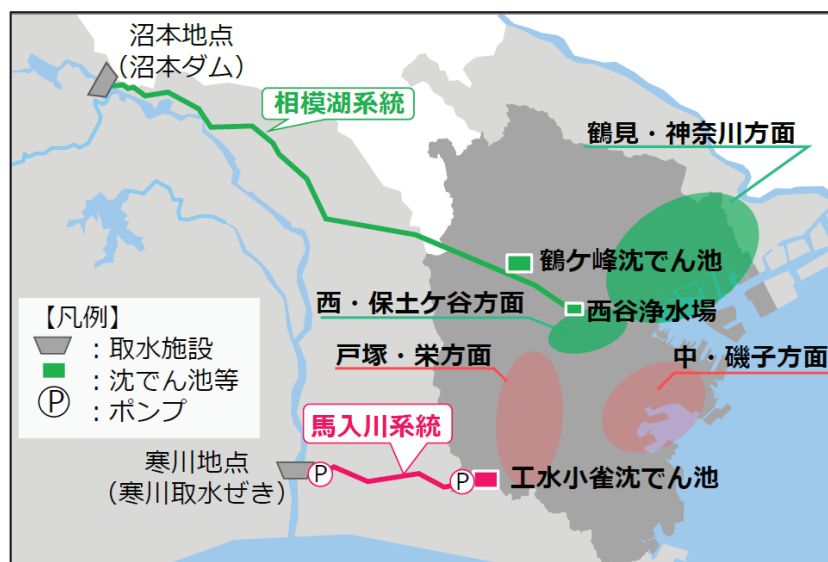
図2-5 工業用水道の施設概要図
