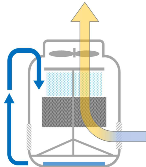
冷却塔の模式図
