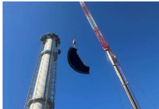
切断した外筒の吊り降ろしの様子
