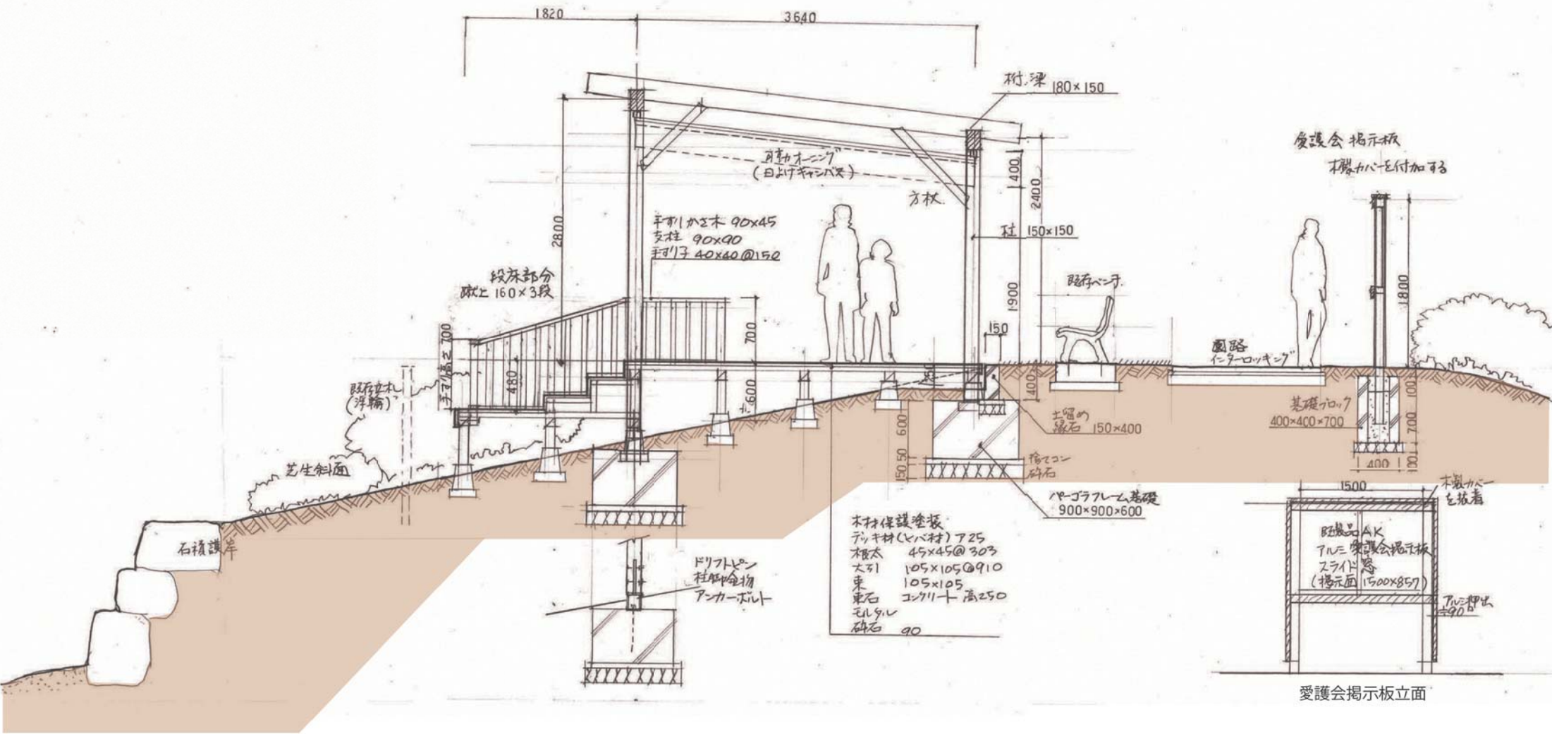
断面図 1:40
