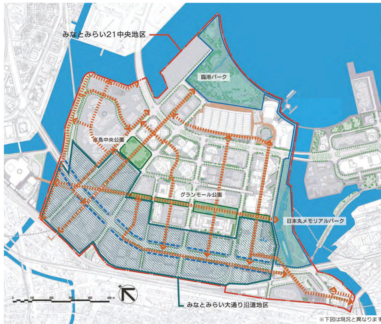
計画図
