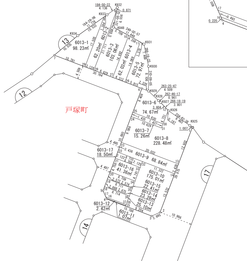
拡大図 1:100
