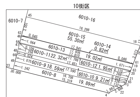
拡大図 1:250
