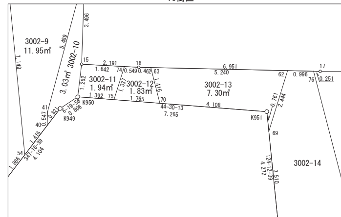
拡大図 1:100
