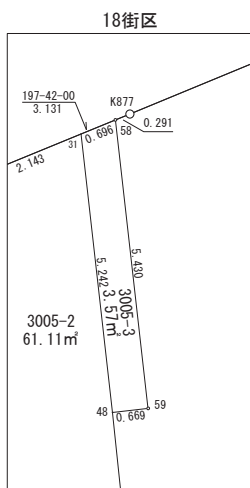
拡大図 1:100
