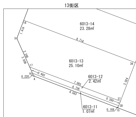
拡大図 1:100
