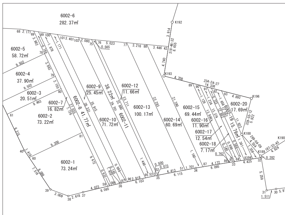
拡大図 1:250
