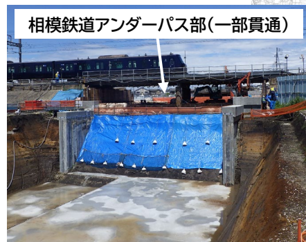
【③瀬谷地内線 アンダーパス部の状況】
