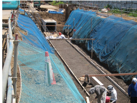
【②下水道工事状況】
