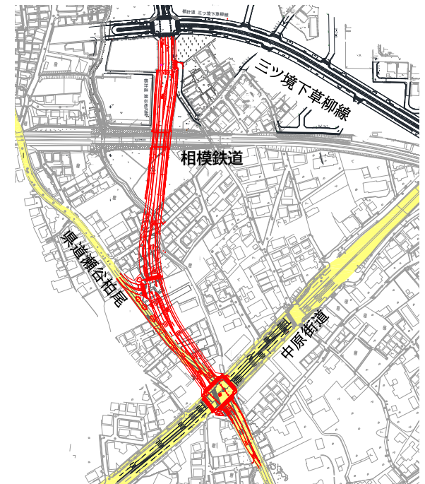
アンダーパス部と擁壁区間のイメージ図
