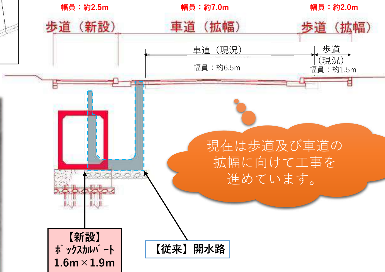
A-A'断面図（イメージ）
