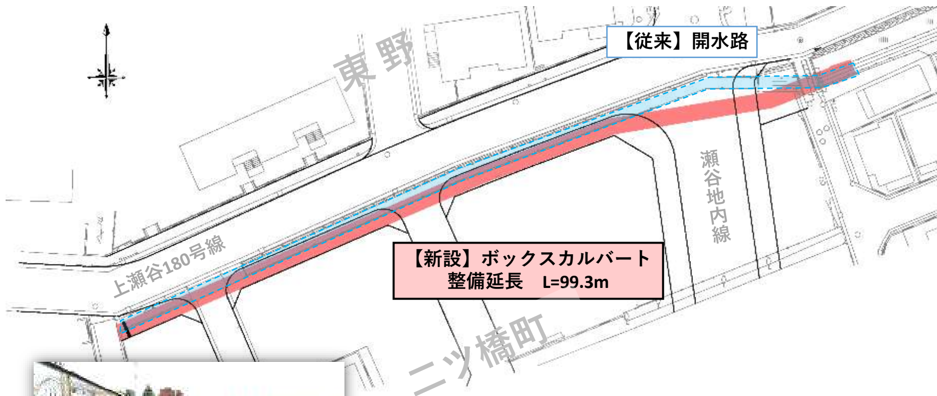
計画平面図
