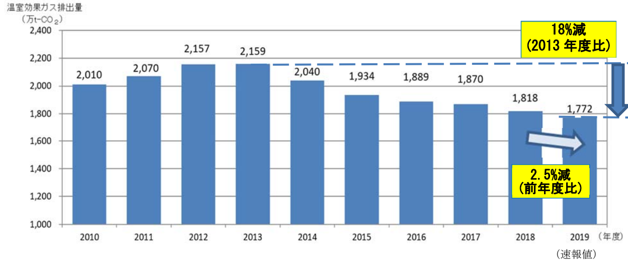
図 1-1 温室効果ガス排出量の経年変化
