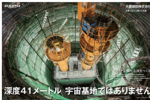
ニューマチックケーソン工事
