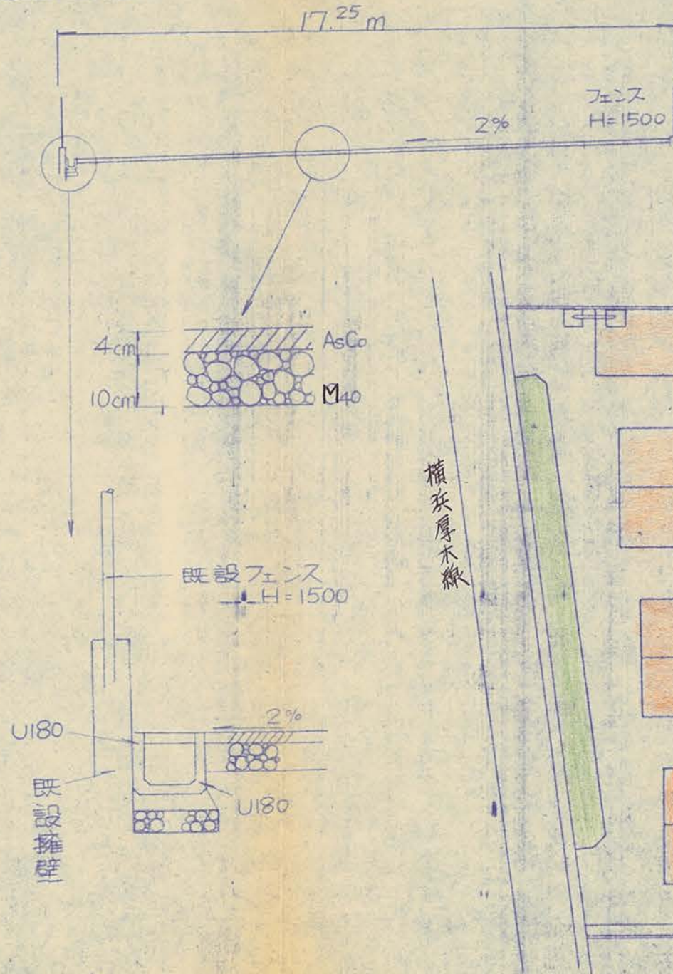
①-① 断面図
