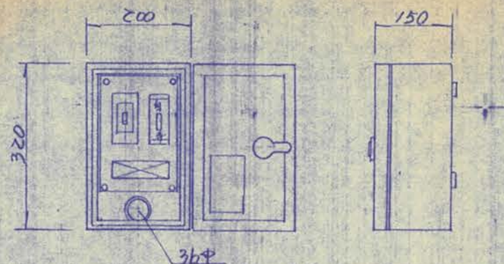
分電盤構造図
