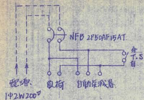
分電盤接続図
