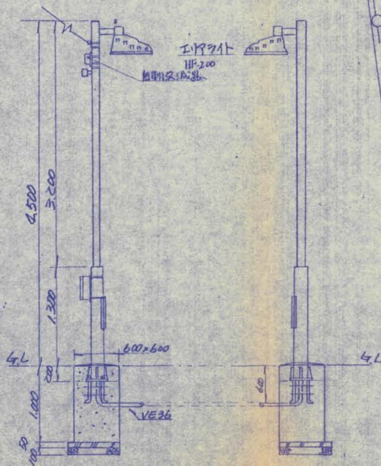
照明柱構造図
