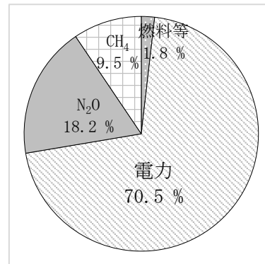
図-1 横浜市西部水再生センターにおけるGHG排出源(令和4年度)
