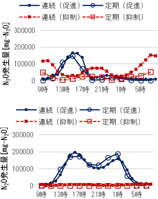
図-3 サンプリング方法ごとの時間帯別 N 2 O 発生量（上段：夏季、下段：秋季）
