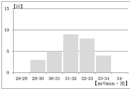
図1 小ブロワ起動時における送風量実績分布 (5月)
