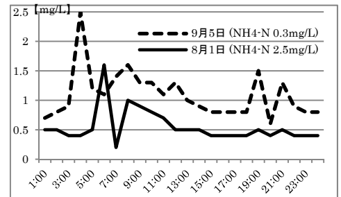
図3 反応タンク DO の日変動
