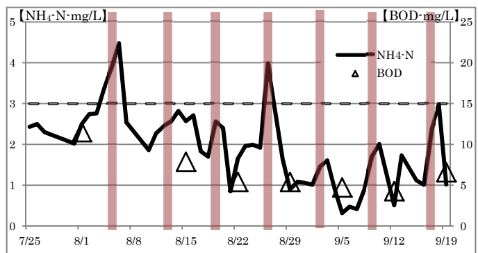
図2 上限設定運転におけるNH 4 -N等の推移 (網掛け縦棒は日曜)
