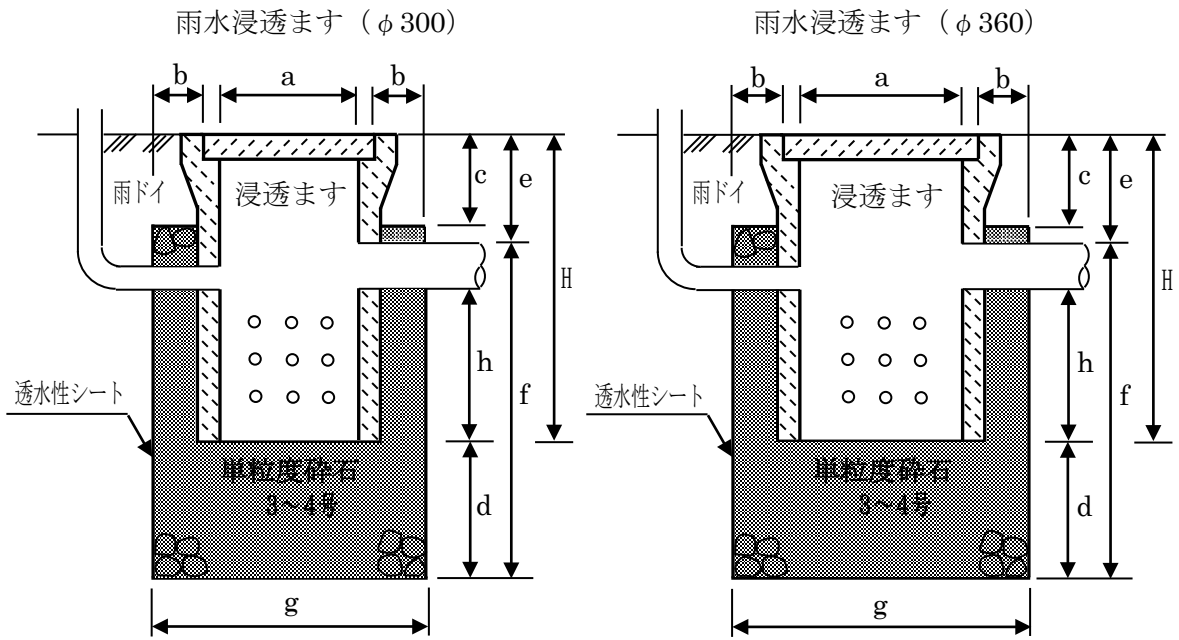
図 3-17 浸透ますの構造図（参考）
