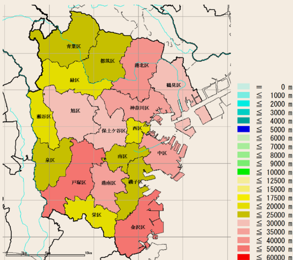
下水管きょ被害延長(m): 元禄型関東地震※
