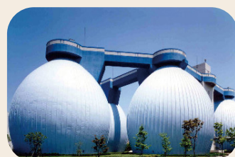
卵形消化タンク
