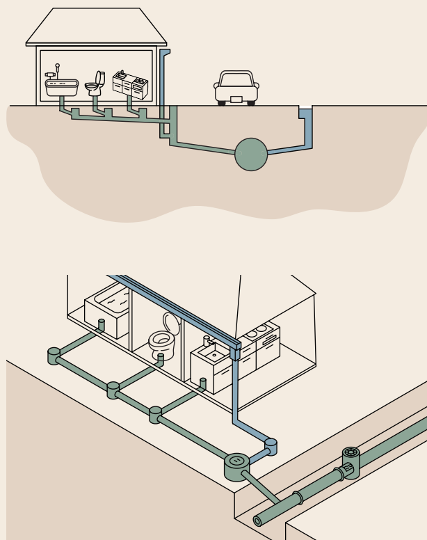
合流式
