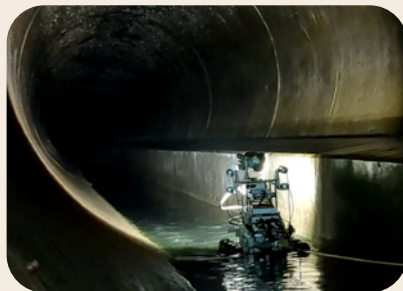
自走式カメラ
