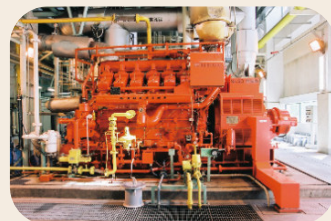
消化ガス発電
