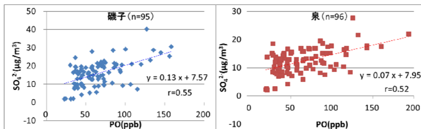
図 10 PO と硫酸イオンとの相関
