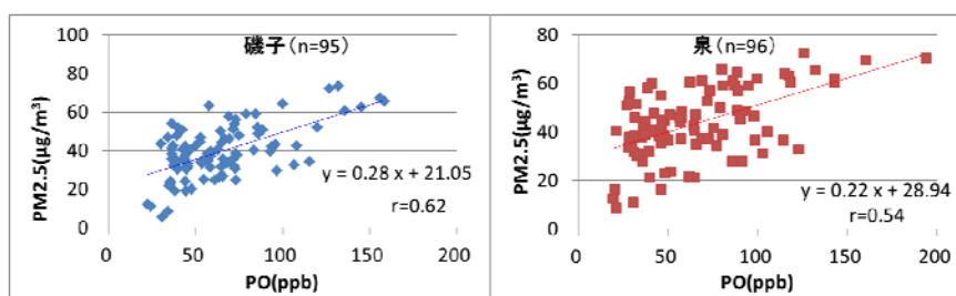
図 9 PO と PM2.5 のとの相関
