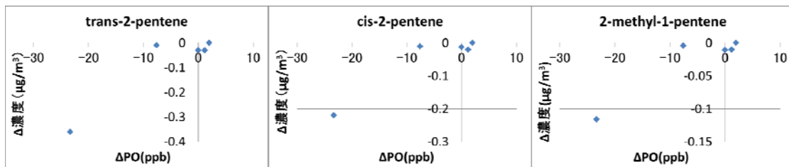
図4 POとVOCとの濃度差の相関
