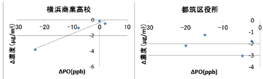
図3 POとホルムアルデヒドとの濃度差の相関
