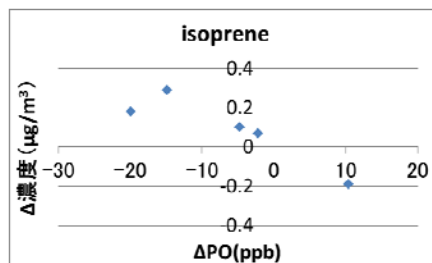
図5 POとVOCとの濃度差の相関
