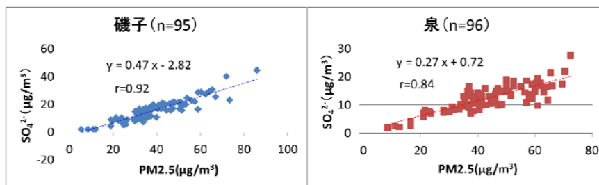
図 8 PM2.5 と硫酸イオンとの相関
