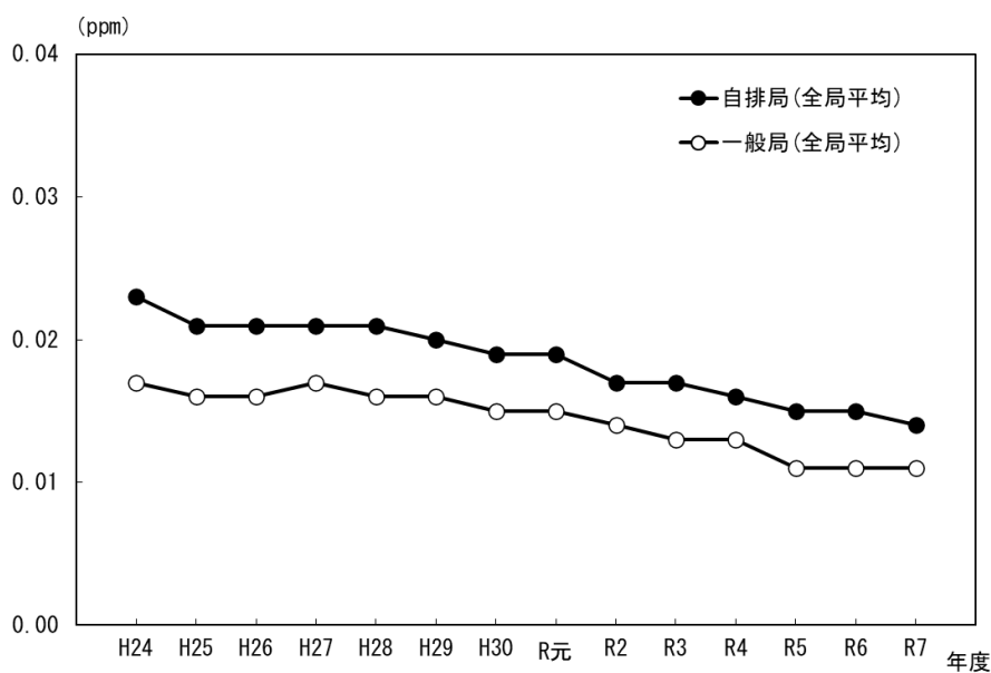
図 2-7 二酸化窒素の年平均値の経年変化
