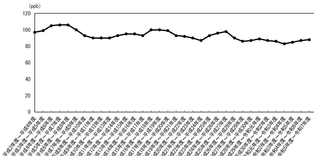
図 2-9 光化学オキシダント濃度の日最高 8 時間値の年間 99 パーセンタイル値の 3 年移動平均値（全測定局）
