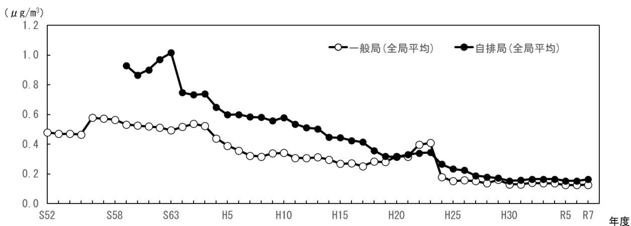
図 2-13 非メタン炭化水素の年平均値の経年変化
