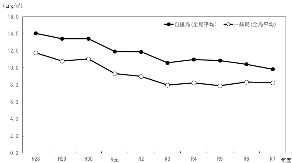
図 2-11 微小粒子状物質の年平均値の経年変化
