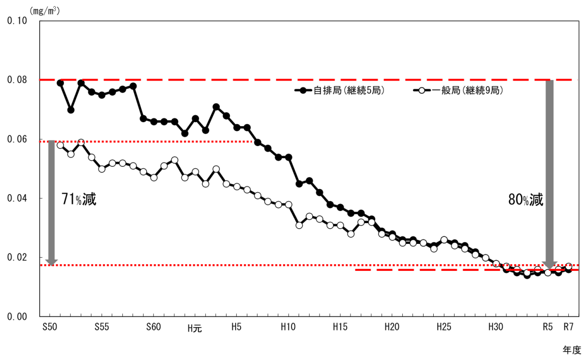
図 2-4 浮遊粒子状物質の年平均値の経年変化（継続測定局）
