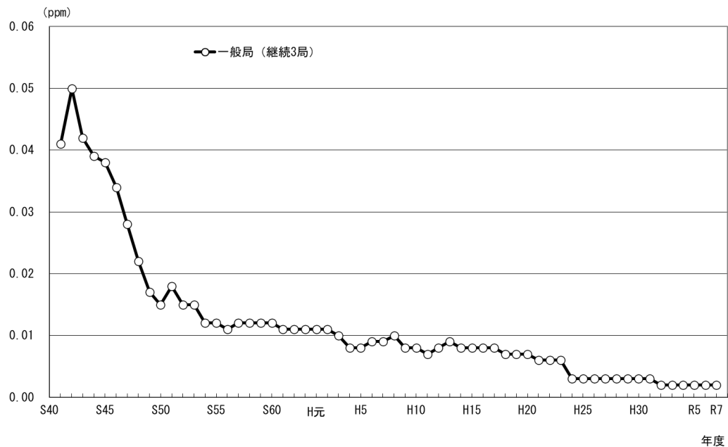
図 2-1 二酸化硫黄の年平均値の経年変化（一般局継続 3 局）
