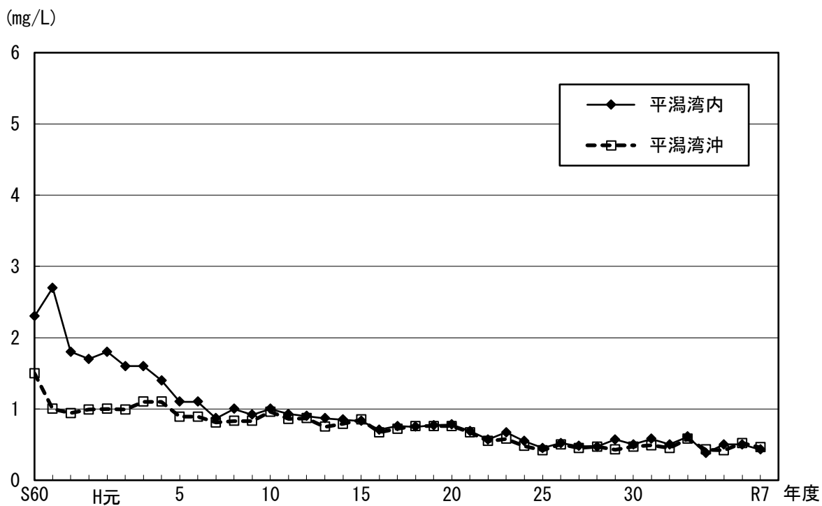
図 2-7 東京湾Ⅲ類型 全窒素年平均値（年度）の経年変化
