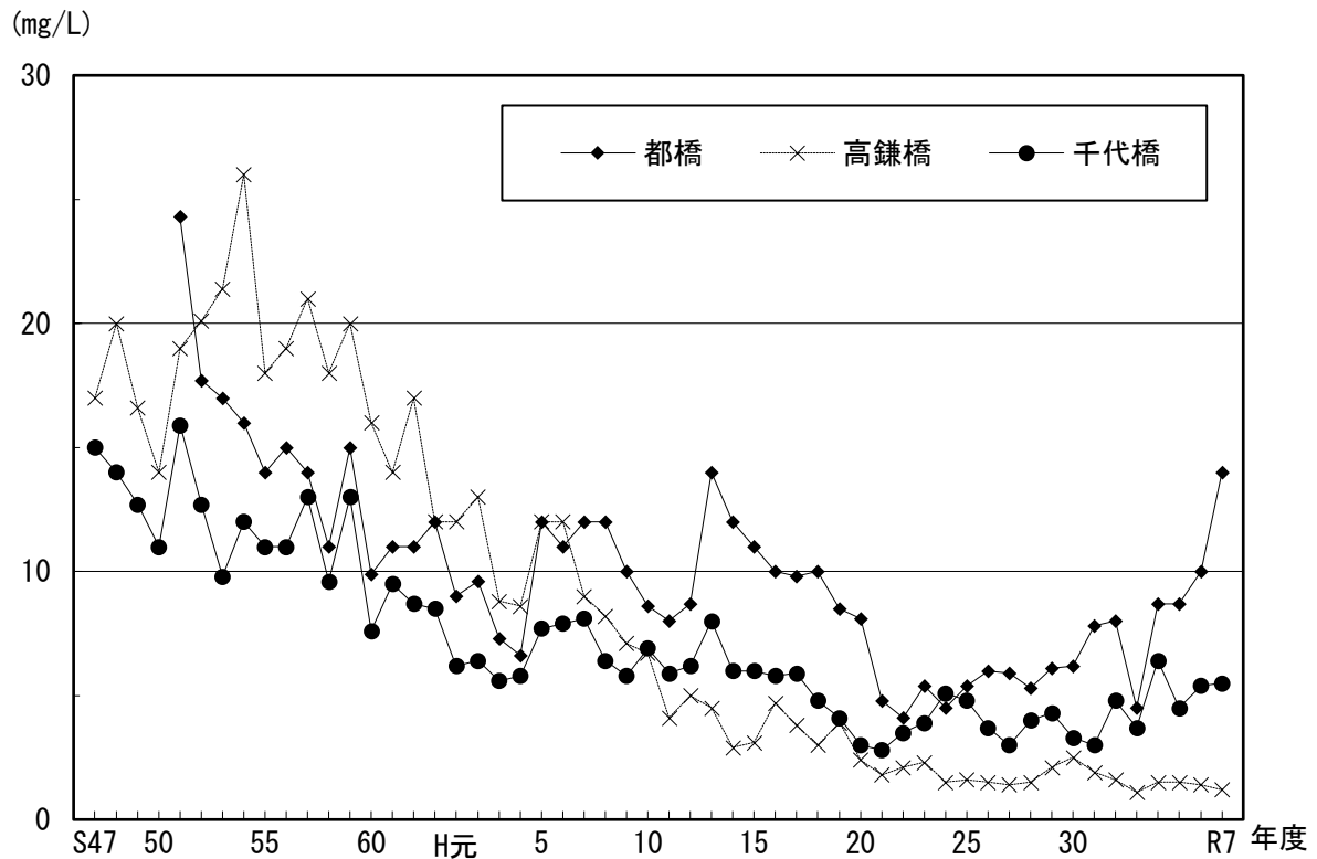
図 2-1 河川 D 類型 BOD 年平均値（年度）の経年変化
