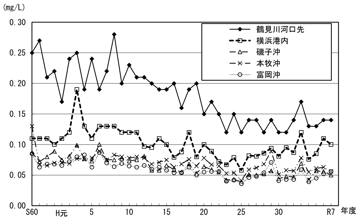
図 2-8 東京湾Ⅳ類型 全燐年平均値（年度）の経年変化
