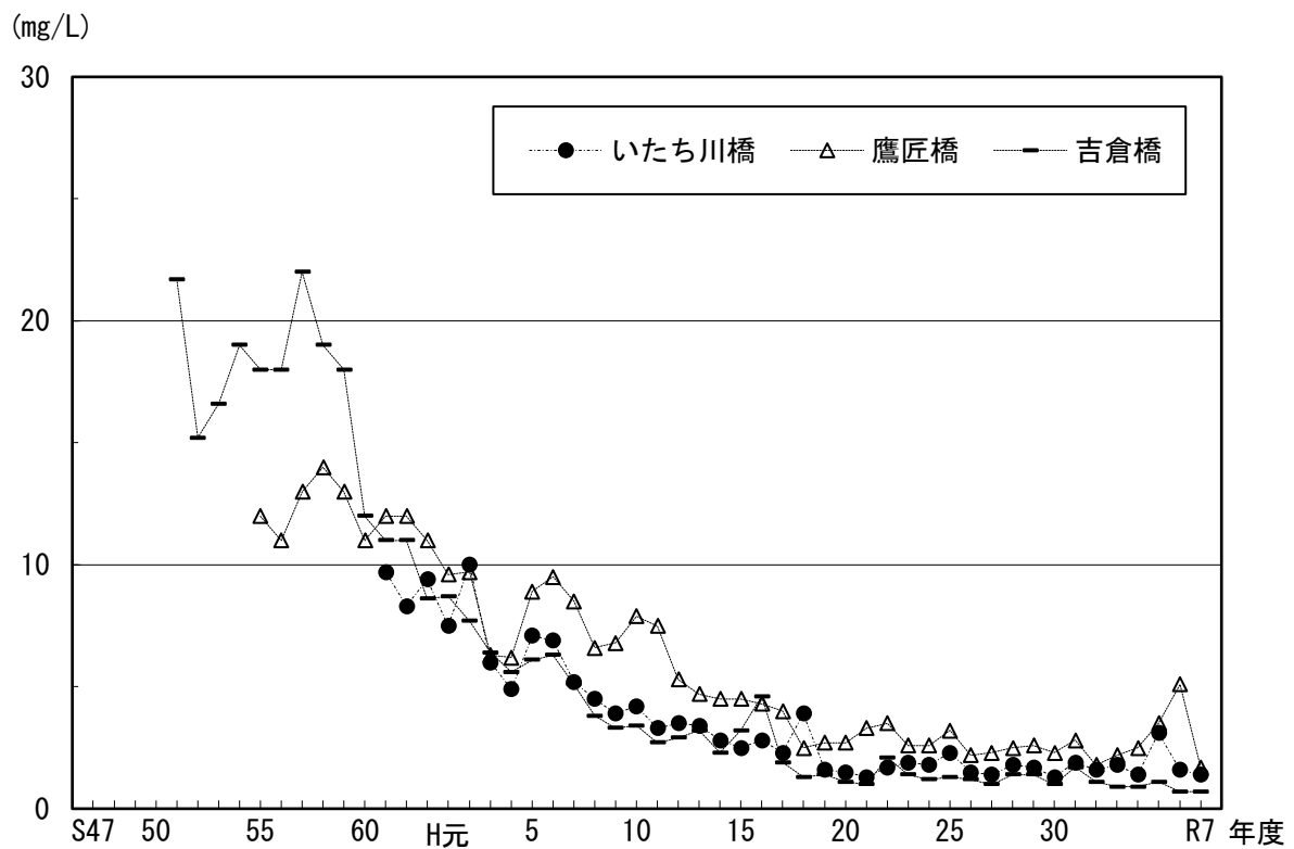
図 2-2 河川 C 類型 BOD 年平均値（年度）の経年変化
