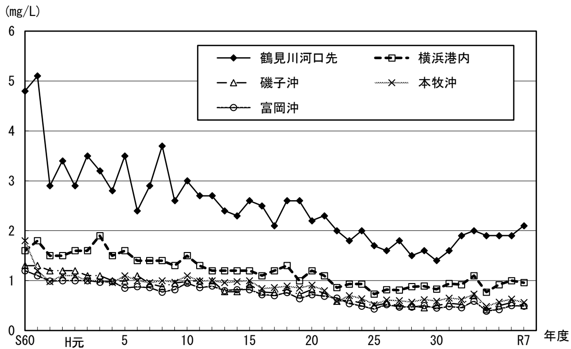
図 2-6 東京湾Ⅳ類型全窒素年平均値（年度）の経年変化
