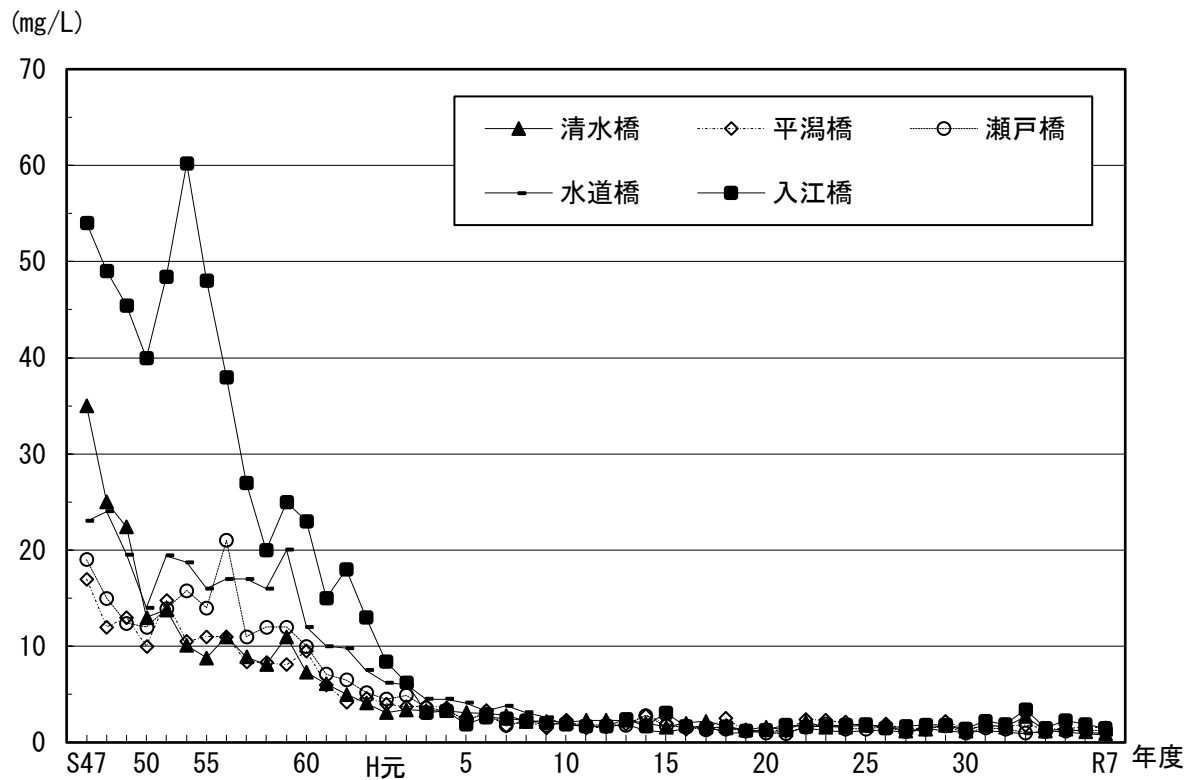
図 2-3 河川 B 類型 BOD 年平均値（年度）の経年変化
