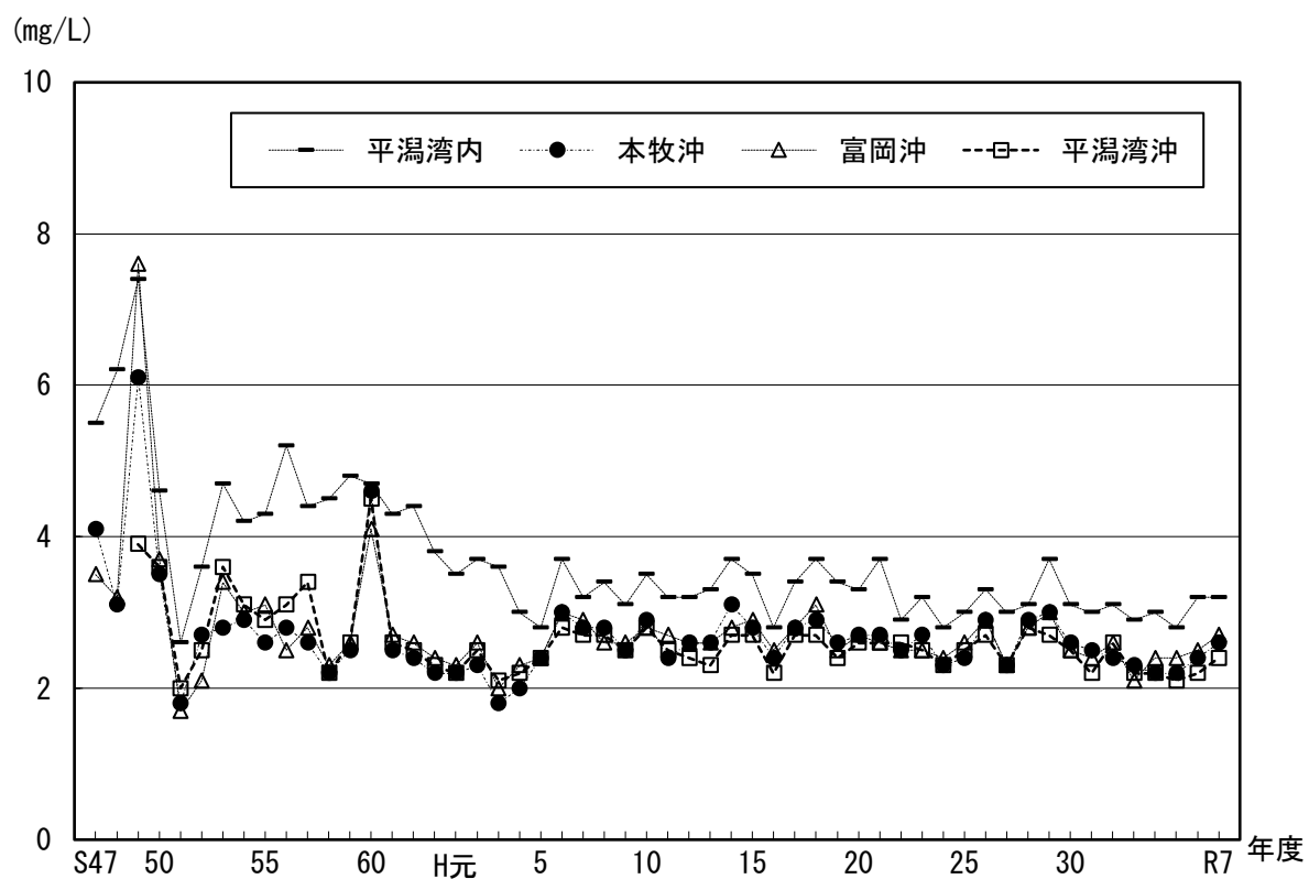
図 2-5 東京湾 B 類型 COD 年平均値（年度）の経年変化
