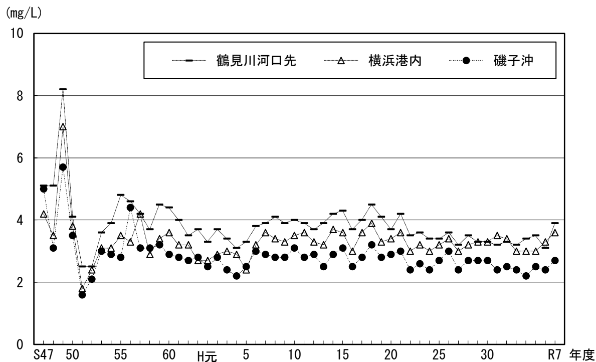
図 2-4 東京湾 C 類型 COD 年平均値（年度）の経年変化
