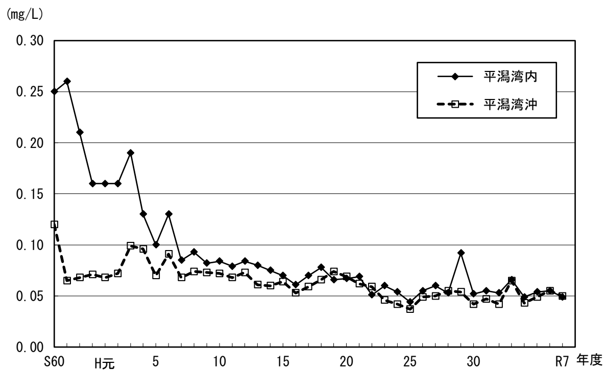
図 2-9 東京湾Ⅲ類型 全燐年平均値（年度）の経年変化
