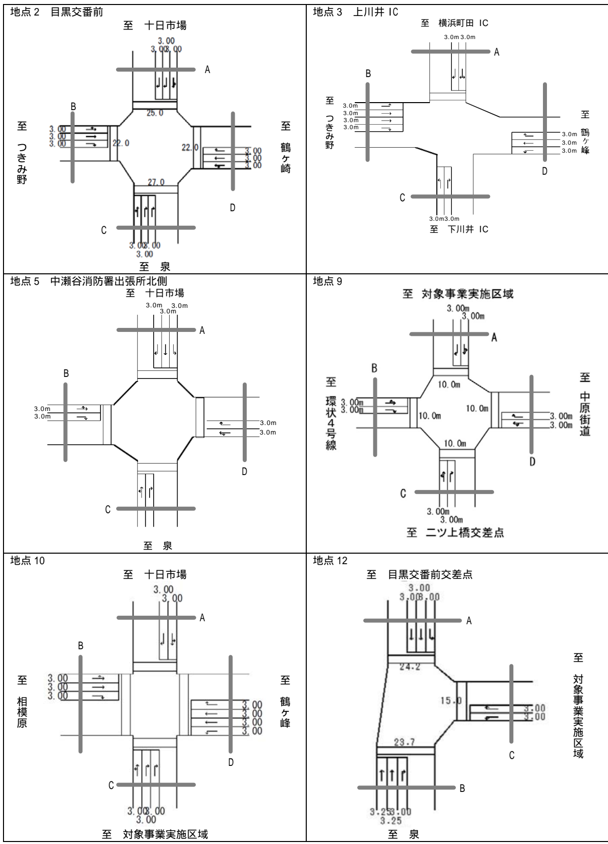
図 6.10-8 将来交差点構造
