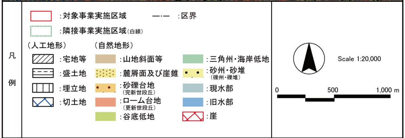
図 3.2-2 地形分類図
