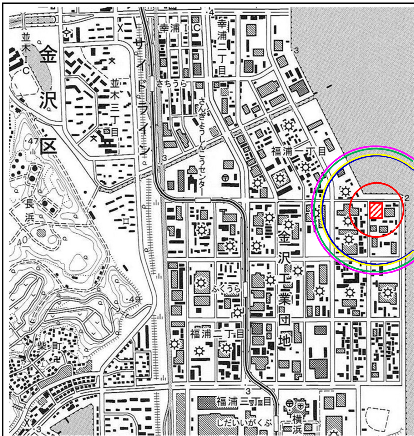
図-6(1) 予測条件別大気質最大着地濃度出現位置(一時間値) 二酸化窒素
