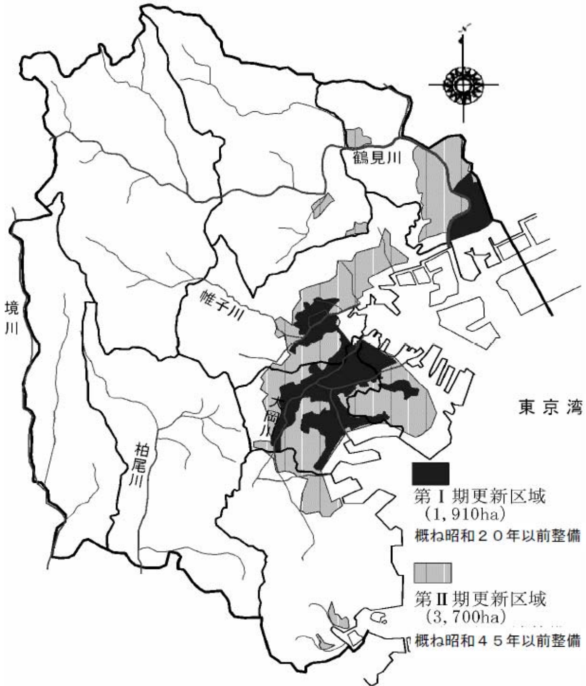
下水道管きよ更新対象区域図
