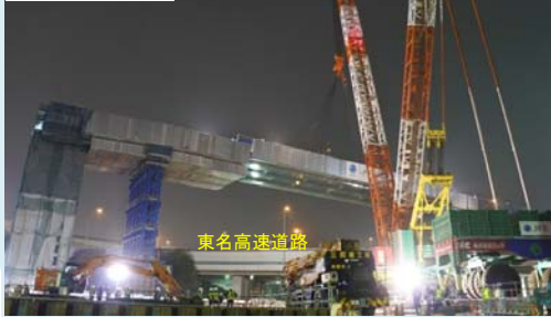
①横浜青葉IC・JCT付近上部工架設(10/11東名通行止め) ※首都高施工区間
