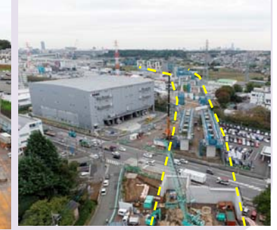
⑨全景 (青葉側から港北方面)
