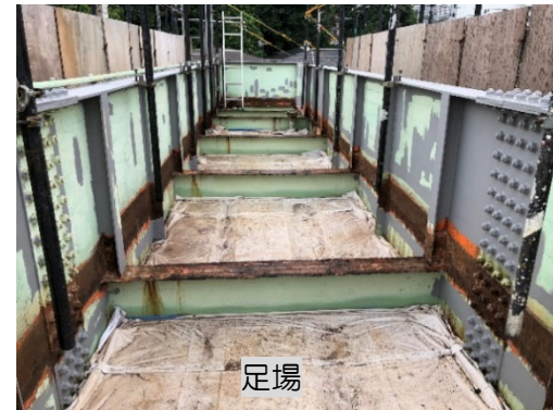
床版・高欄撤去時の様子（市内補修事例より）
