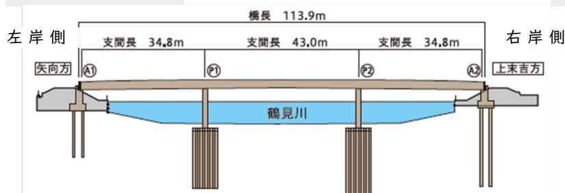
【側面図】
