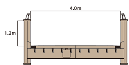
【断面図】
