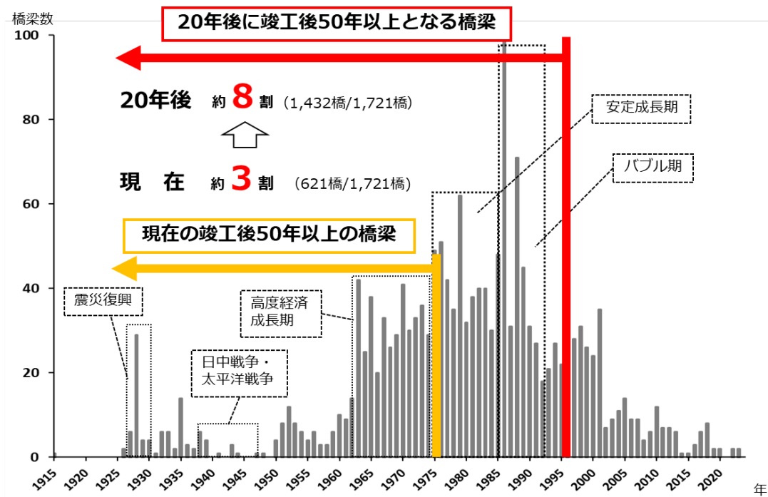
図3 横浜市管理橋梁の竣工年の現状
