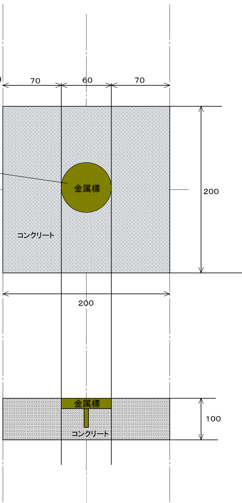
二次節点 構造図 (mm)
