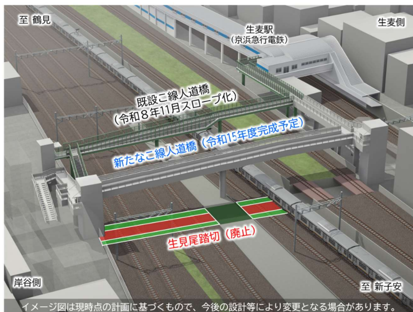
新たなこ線人道橋イメージ (令和15年度完成予定)
