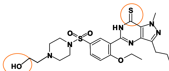
図1 ヒドロキシチオホモシルデナフィルの化学構造式
