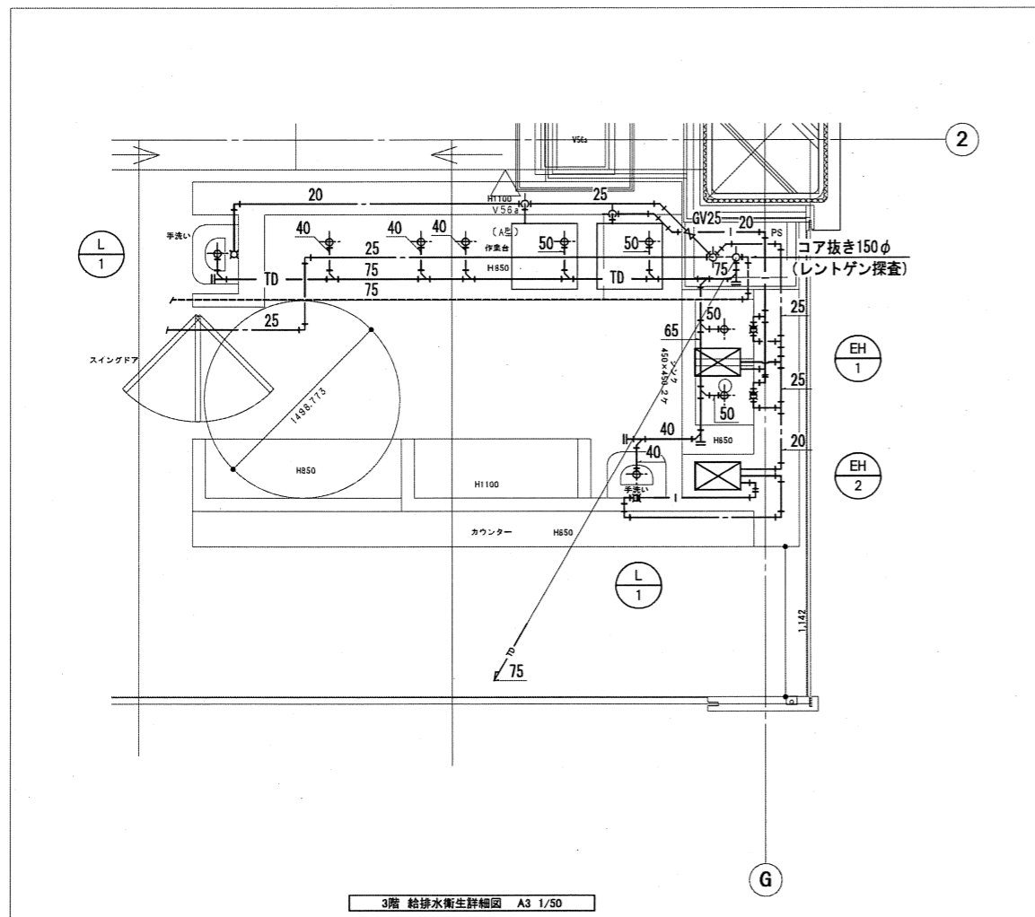
3階 給排水衛生詳細図 A3 1/50
