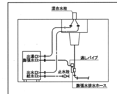
電気温水器配管要領図
