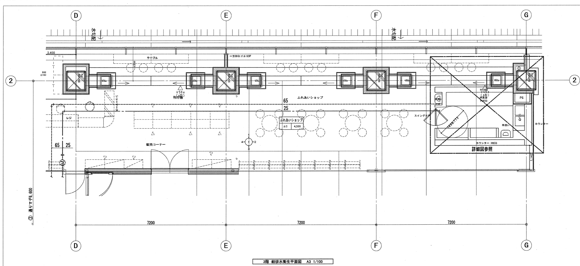
3階 給排水衛生平面図 A3 1/100
